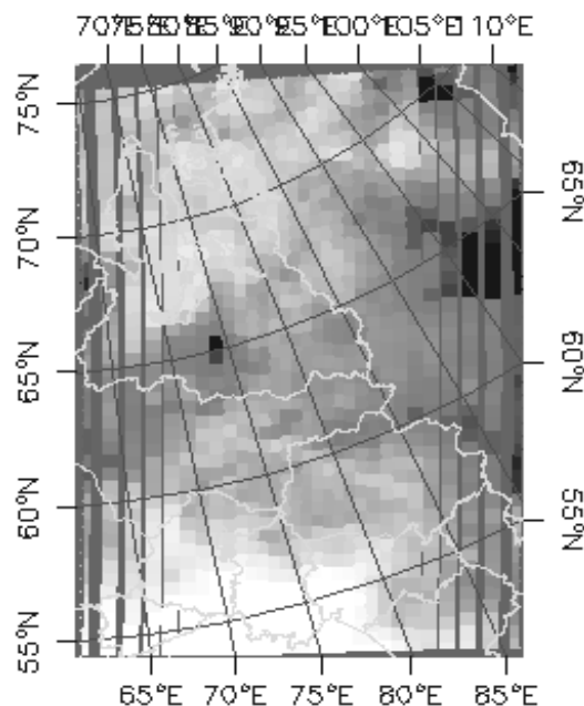
Рис. 1. Геопривязанный кадр AMSU на 29.02.2012 г., частота 23 ГГц, с наложенными границами субъектов РФ
